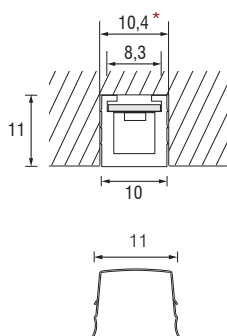
Clip di fissaggio (opzionali)
