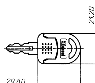
CHIAVE A SNODO - HINGED KEY
