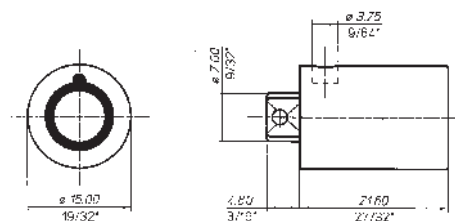
Nucleo con foro per spinatura Nucleo with fixing hole
