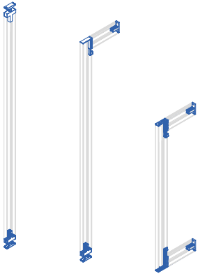
Mounting structure I (floor - ceiling) Konstrukcja montażowa I (podłoga - sufit)
