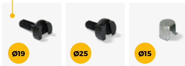
Insert fastener Zaczep klinowy
