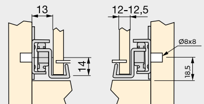
C - Sockets \text{Ø}8 \times 8 /C - Gniazda \text{Ø}8 \times 8
