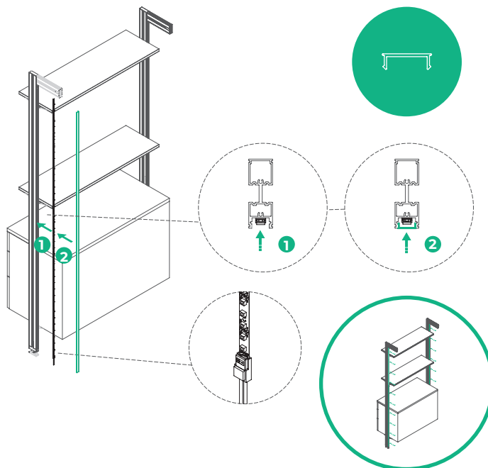
Illuminazione superiore Superior lighting
