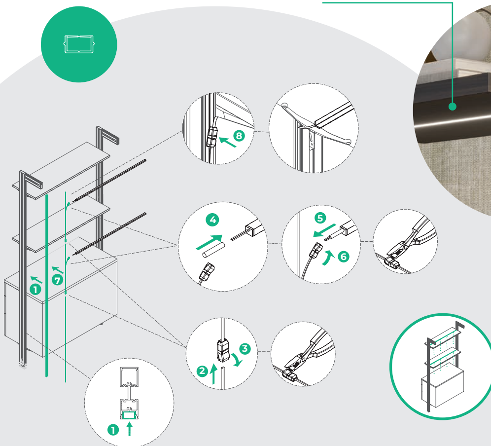
Illuminazione superiore Superior lighting
