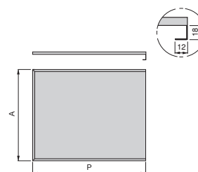
Fondi sotto lavello 18mm Base plate protectors 18 mm
