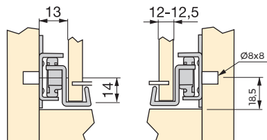
C - A pressione Ø8x8/C - Knock-in Ø8x8
