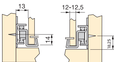
C - Per vite/C - Screw-on
